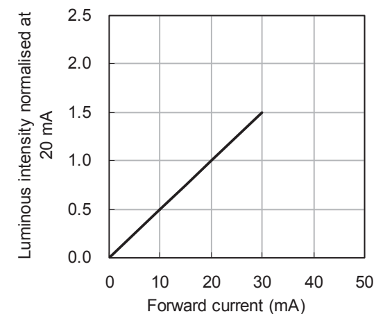
相对光强与电流特性曲线 Luminous Intensity vs. Forward Current
