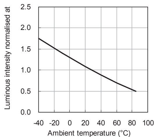
相对光强与环境温度特性曲线 Luminous Intensity vs. Ambient Temperature
