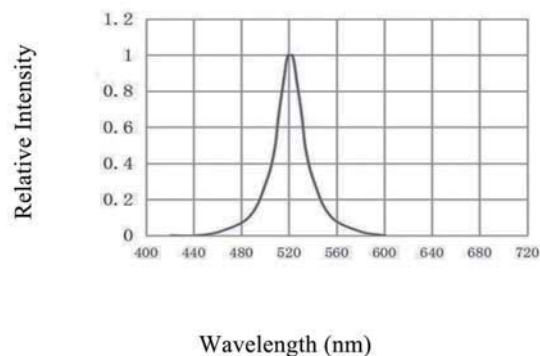
光谱分布特性曲线 Spectrum Distribution ( T_a=25^\circ\text{C} )
