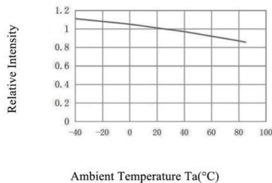
相对光强与环境温度特性曲线 Relative Intensity VS. Ambient Temperature ( T_a=25^\circ\text{C} )
