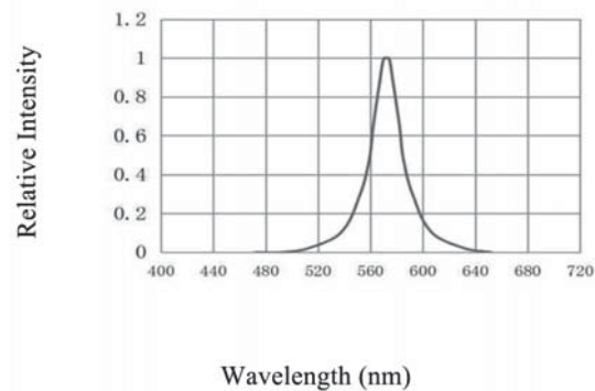
光谱分布特性曲线 Spectrum Distribution (Ta=25°C)
