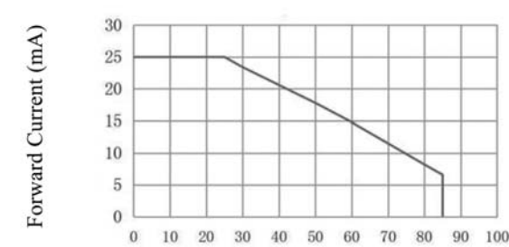
最大正向电流与环境温度特性曲线 Maximum Forward Current VS. Ambient temperature
