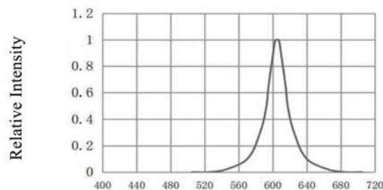
光谱分布特性曲线 Spectrum Distribution (Ta=25°C)
