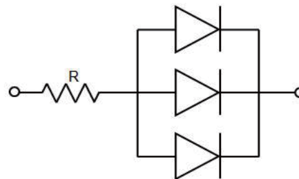
电路模式/ Circuit model B
