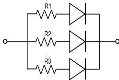
电路模式/ Circuit model A
