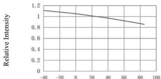
相对光强与环境温度特性曲线 Relative Intensity VS. Ambient Temperature (Ta=25°C)
