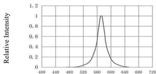
光谱分布特性曲线 Spectrum Distribution (Ta=25°C)
