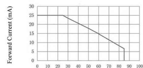
最大正向电流与环境温度特性曲线 Maximum Forward Current VS. Ambient temperature
