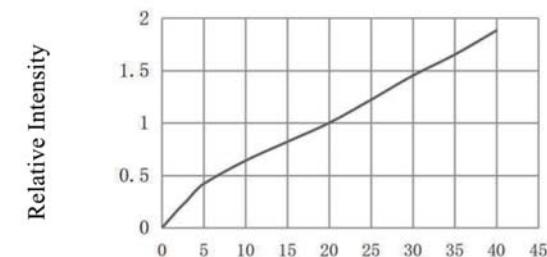
相对光强与电流特性曲线 Relative Intensity VS. Forward Current (Ta=25°C)
