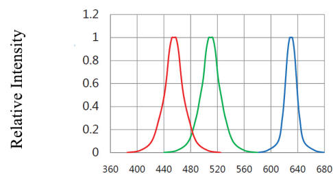
光谱分布特性曲线 Spectrum Distribution (Ta=25°C)
