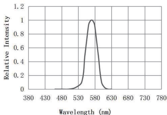
光谱分布特性曲线 Spectrum Distribution (Ta=25°C)
