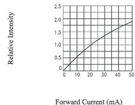
相对光强与电流特性曲线 Relative Intensity VS. Forward Current (Ta=25°C)
