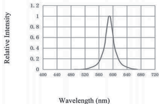
光谱分布特性曲线 Spectrum Distribution (Ta=25°C)
