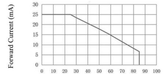
最大正向电流与环境温度特性曲线 Maximum Forward Current VS. Ambient temperature
