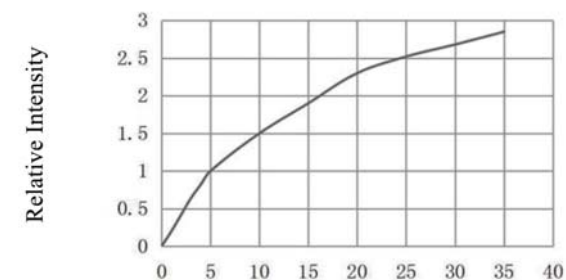
相对光强与电流特性曲线 Relative Intensity VS. Forward Current (Ta=25°C)
