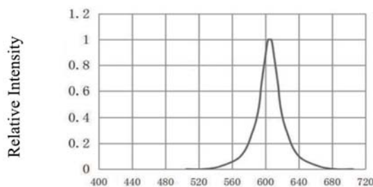
光谱分布特性曲线 Spectrum Distribution (Ta=25°C)
