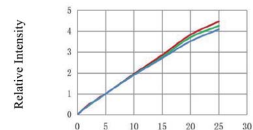
相对光强与电流特性曲线 Relative Intensity VS. Forward Current (Ta=25°C)
