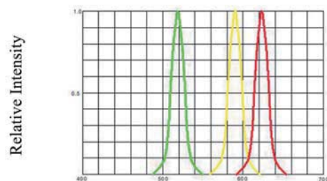
光谱分布特性曲线 Spectrum Distribution (Ta=25°C)
