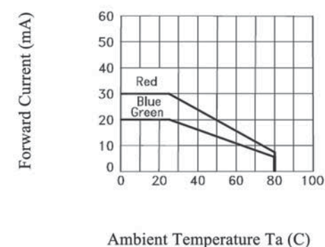
最大正向电流与环境温度特性曲线 Maximum Forward Current VS. Ambient temperature
