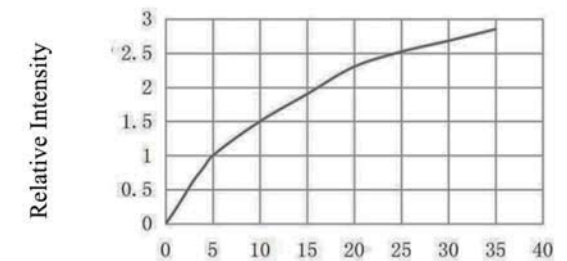
相对光强与电流特性曲线 Relative Intensity VS. Forward Current (Ta=25°C)
