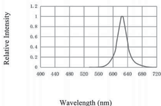
光谱分布特性曲线 Spectrum Distribution (Ta=25°C)
