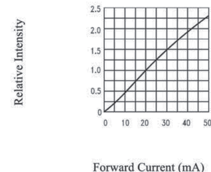
相对光强与电流特性曲线 Relative Intensity VS. Forward Current (Ta=25°C)
