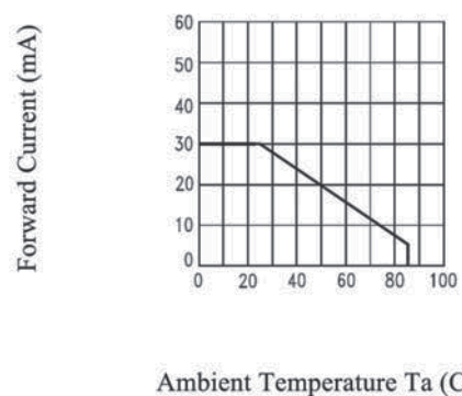
最大正向电流与环境温度特性曲线 Maximum Forward Current VS. Ambient temperature
