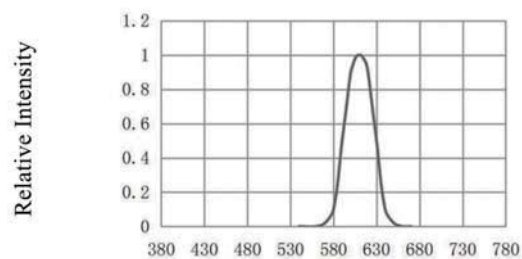
光谱分布特性曲线 Spectrum Distribution (Ta=25°C)
