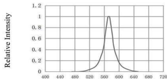
光谱分布特性曲线 Spectrum Distribution (Ta=25°C)
