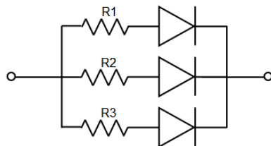
电路模式/ Circuit model A
