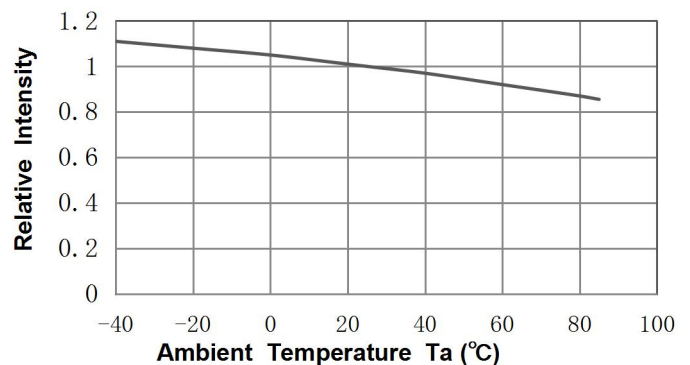
相对光强与环境温度特性曲线 Relative Intensity VS. Ambient Temperature ( T_a=25^{\circ}\text{C} )
